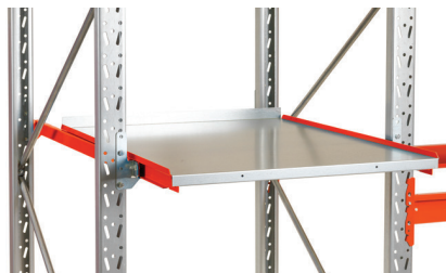
Výsuvná police se spodním platem pro pohodlné vychystávání nepaletizovaného zboží - instalace na regálových stojinách nebo na příčném nosníku (vyšší nosnost).
